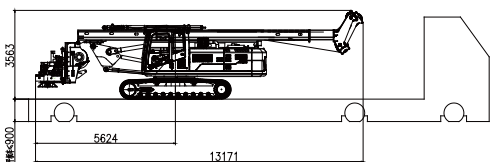
不带钻杆运输状态
