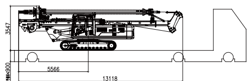
带8米钻杆运输状态
