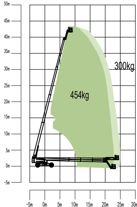
ZT42JEH 作业曲线图
