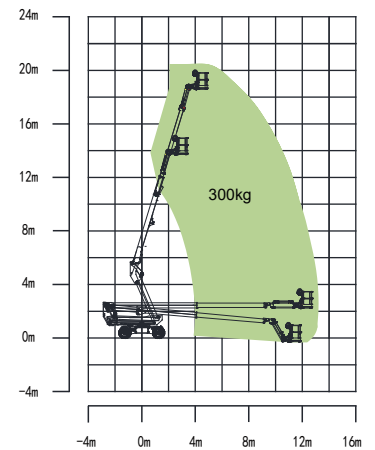
ZT18JE/ZT18JE-Li 作业曲线图
