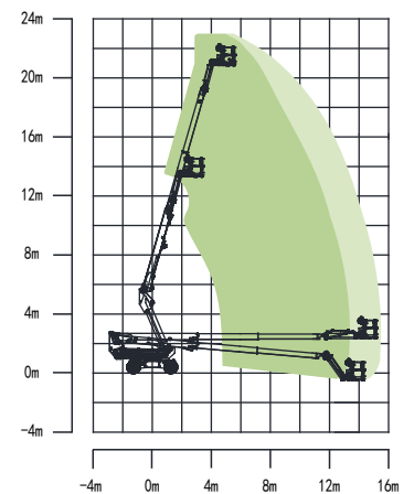
ZT21JE/ZT21JE-Li 作业曲线图
