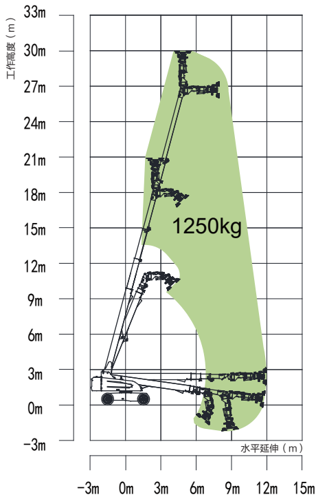
ZTV30-1250作业曲线图
