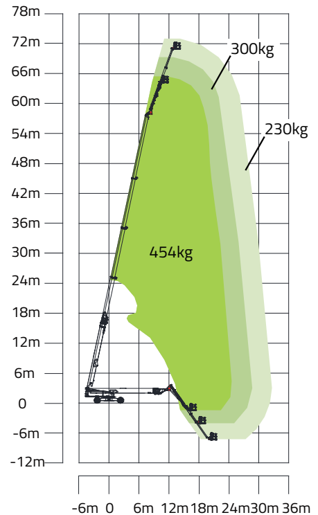
ZT72J作业曲线图
