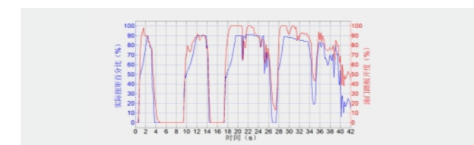
整车与底盘动力匹配曲线
