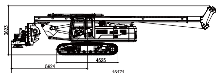
不带钻杆运输状态
