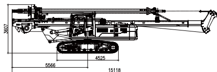
带10米钻杆运输状态
