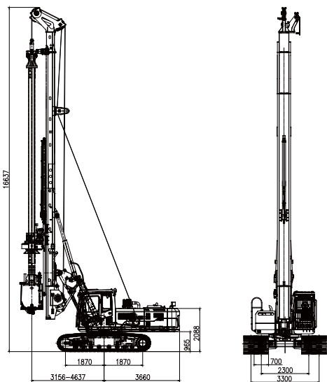
其中3156-3500范围可用于钻孔作业 去除钻杆钻具
