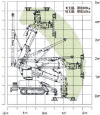
SR-V800 作业曲线图
