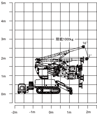
SR-V800 吊装工作曲线图
