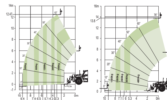
ZTH4014作业曲线图
