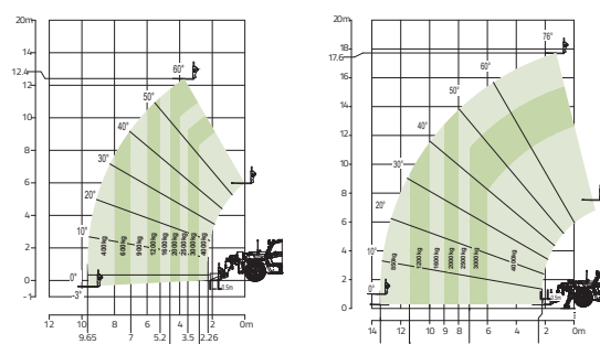
ZTH4018作业曲线图
